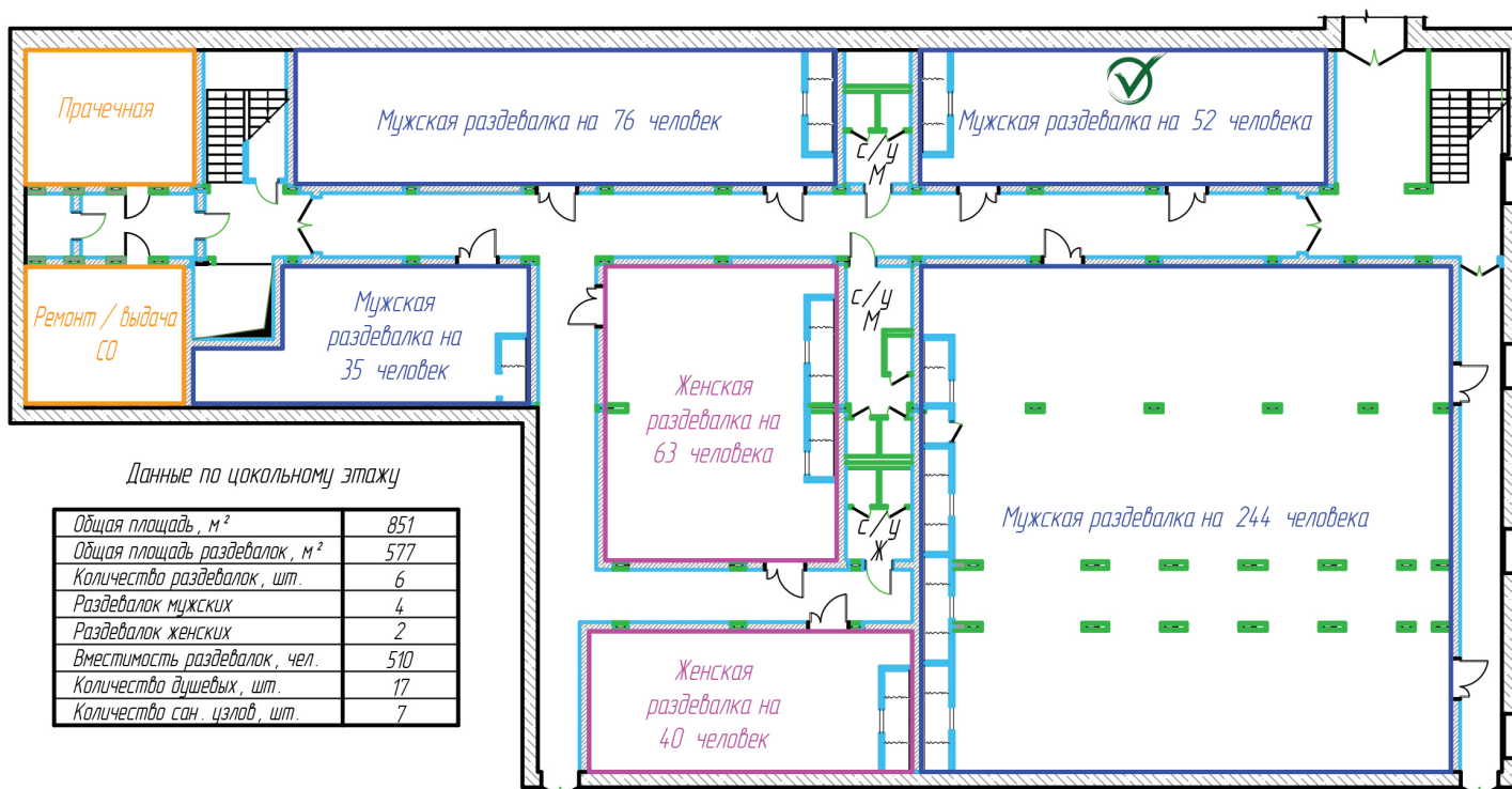
План -1 этажа административно-бытового комплекса
